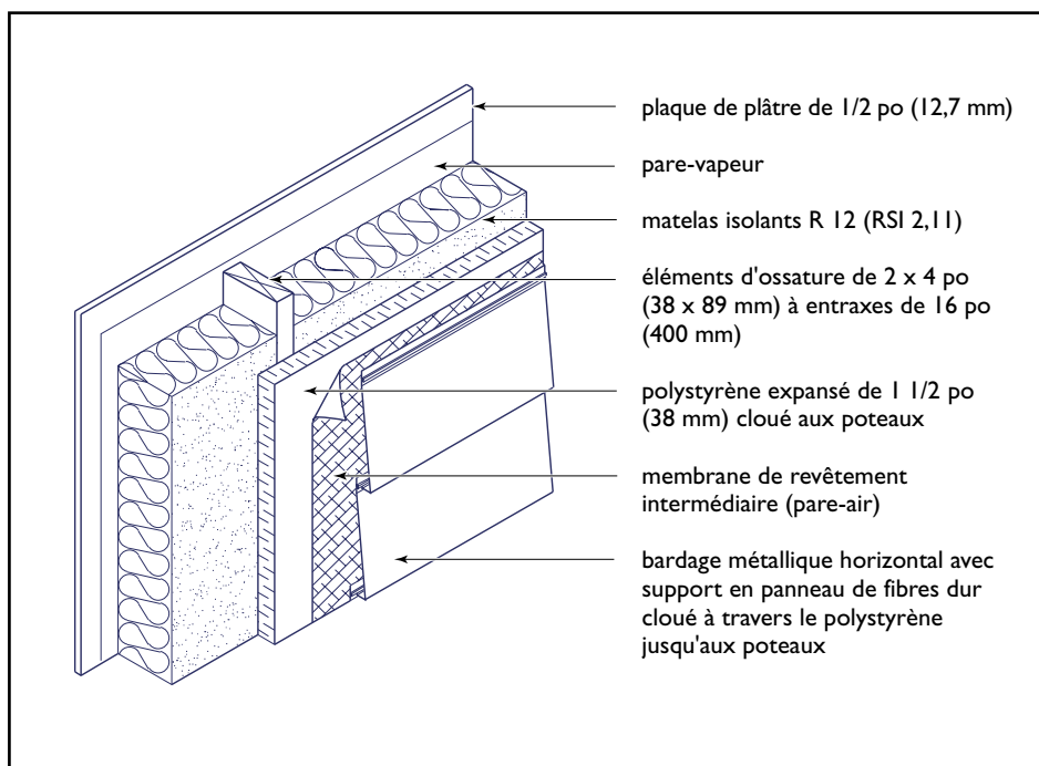
Figure 1 Valeur de résistance thermique effective : R 16,7 (RSI 2,94)
